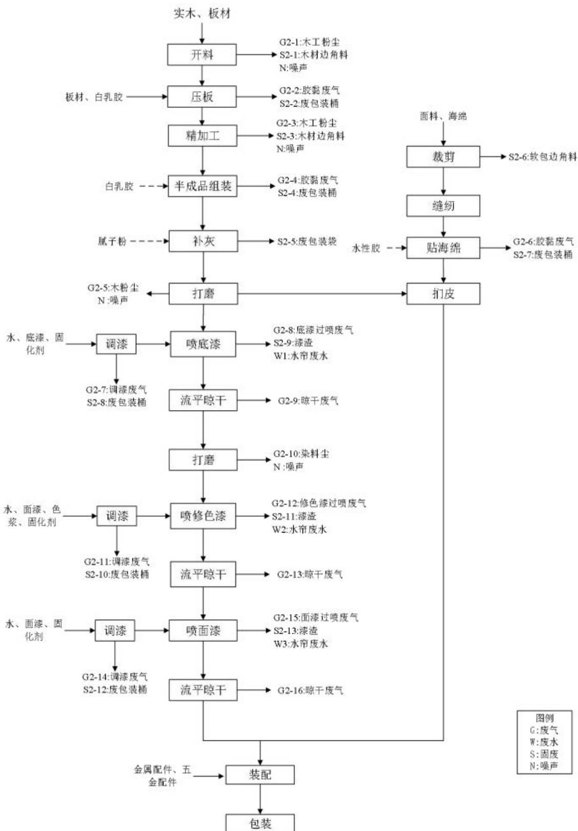
图 1-3-2 生产工艺流程图（家具生产）
